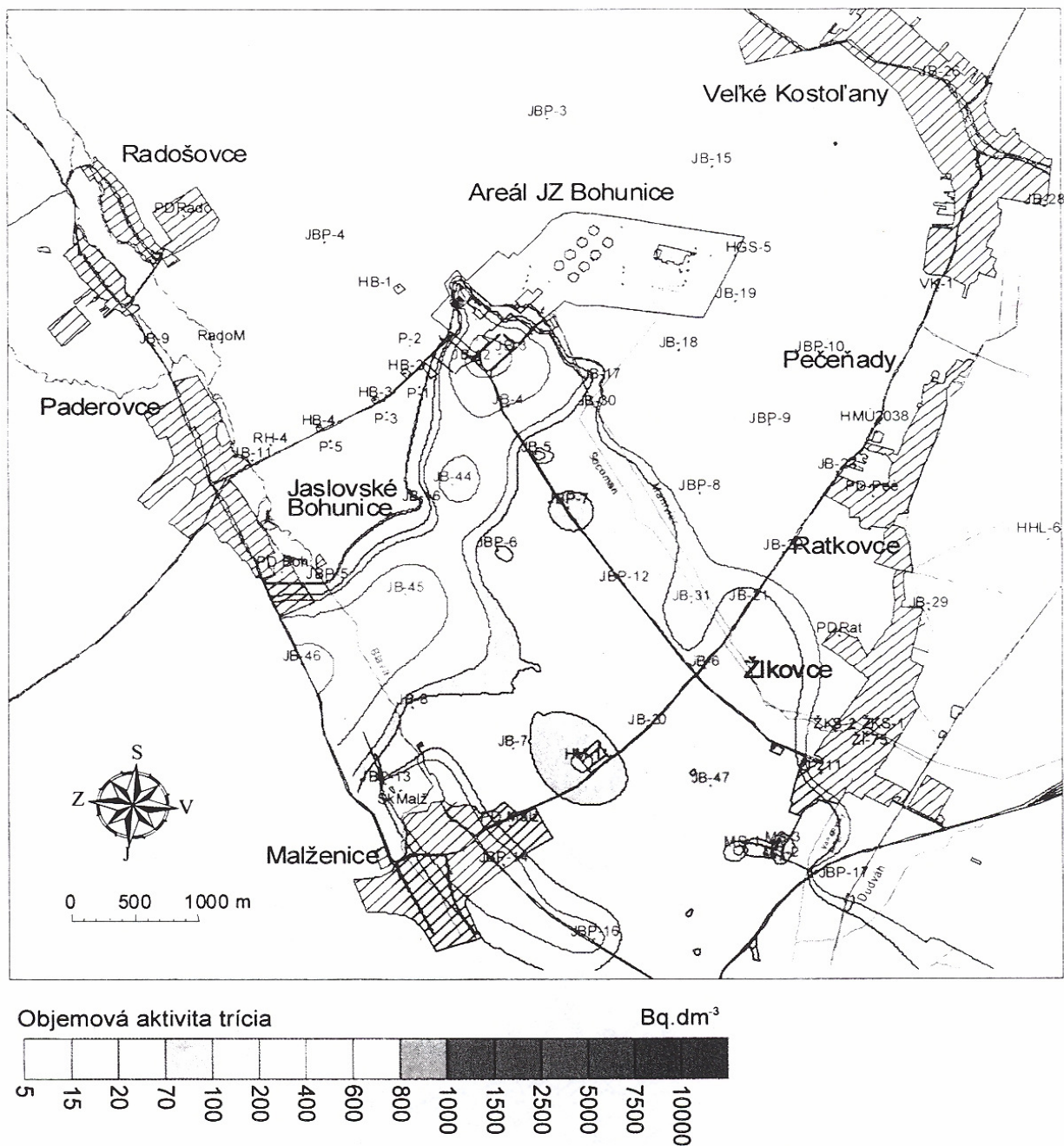
Abb. 6 Isolinien der Volumenaktivität von Tritium im Grundwasser in der weiteren Umgebung území (Stand August 2005)
